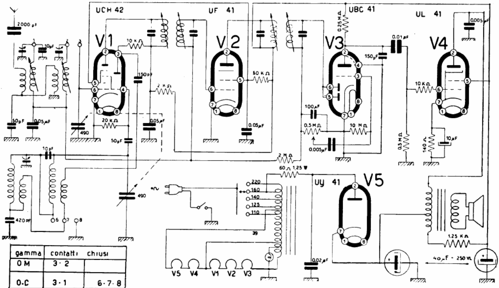
VEGA - Modd. 527 serie ANIE e 529. Onde medie da 520 a 1620 kc/s. Onde corte da 5,8 a 18,1 Mc/s. Media frequenza 470 kc/s. Potenza indistorta di uscita 1,5 watt. Consumo 28 watt.
